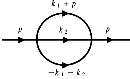
FIG. 1. Sunset diagram.
